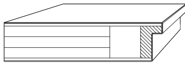
TYP 50, TÜRDICKE CA. 50 MM Feuerschutztür T30(EI30) Rauchschutztür RS(S200) Einbruchhemmende Tür RC2 Schallschutztür SK32/2 Schallschutztür SK37/3
