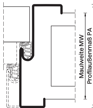
Stumpf/stumpf mit Leibungsfalz
