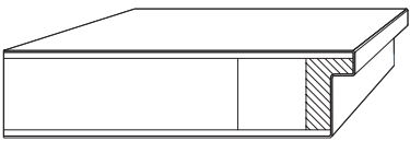
TYP 50, TÜRDICKE CA. 50 MM Vollspanplattentür Feuerschutztür T30(EI30) Rauchschutztür RS(S200) Einbruchhemmende Tür RC2 Schallschutztür SK27/1
